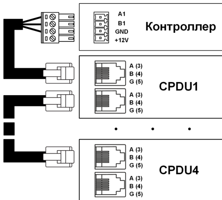
Рис. 3. Схема подключения CPDU
