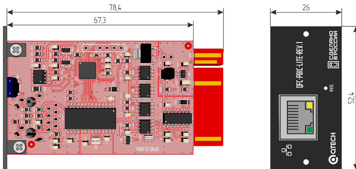
Рисунок 1. QFC-PBIC-LITE-REV.1
